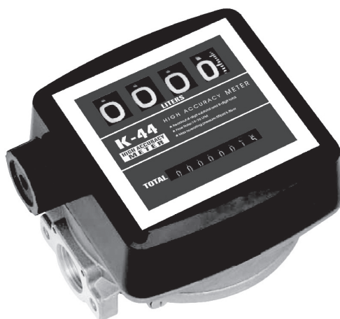
2. ZÄHLWERK FÜR EXELENZ 2.1, MECHANISCH (DPY01108-4)
